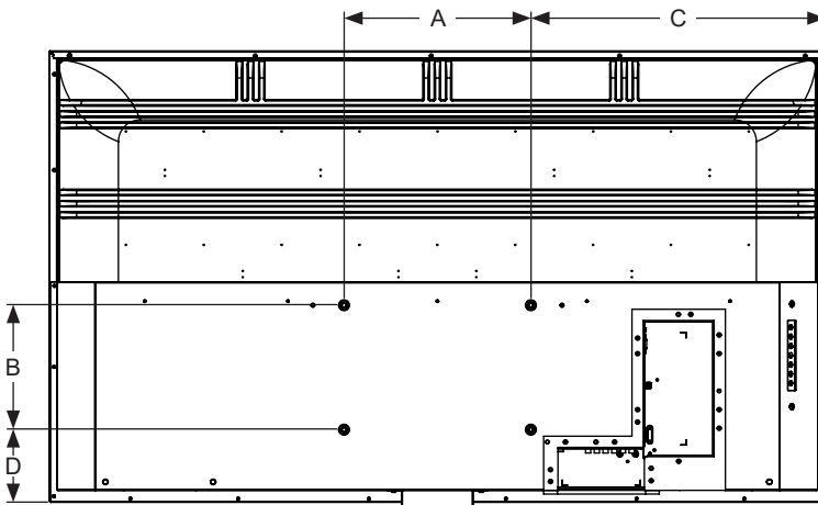
VISTA TRASERA
