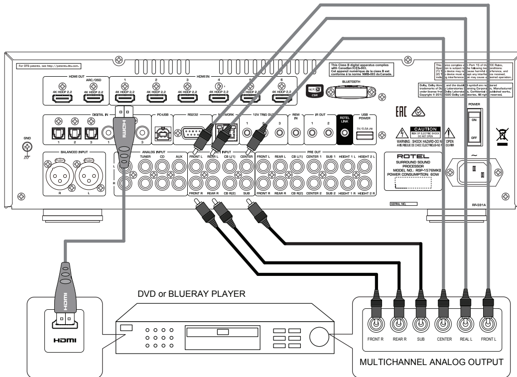
Figure 5: Blu-Ray and Video Player Connections Connexions à un lecteur Blu-Ray ou Vidéo Anschlussdiagramm für Blu-Ray- und Video-Player Conexiones para Reproductor de Video o Blu-Ray
