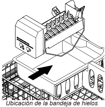
Ubicación de la bandeja de hielos
