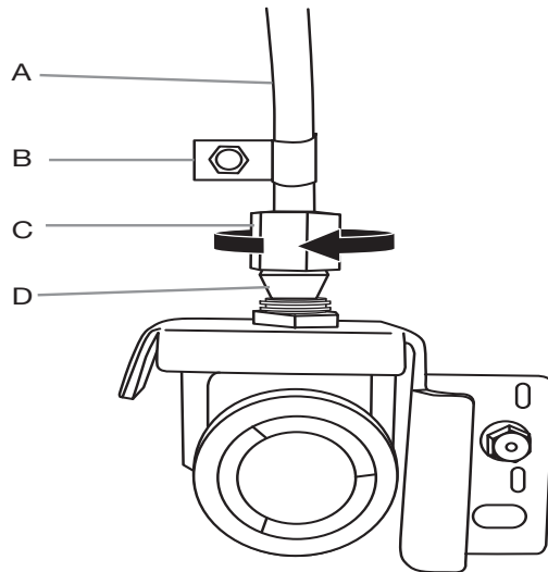
A. Copper tubing B. "P" clamp
