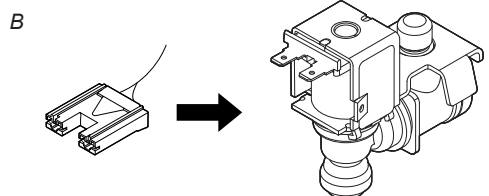
Raccorder le bon connecteur de faisceau à l'électrovanne
