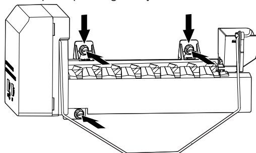
Mantenga las perchas contra los tornillos mientras aprieta
