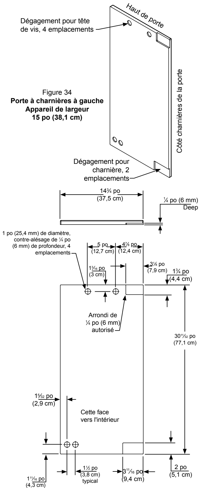
Figure 35 Porte à charnières à gauche Appareil de largeur 15 po (38,1 cm)
