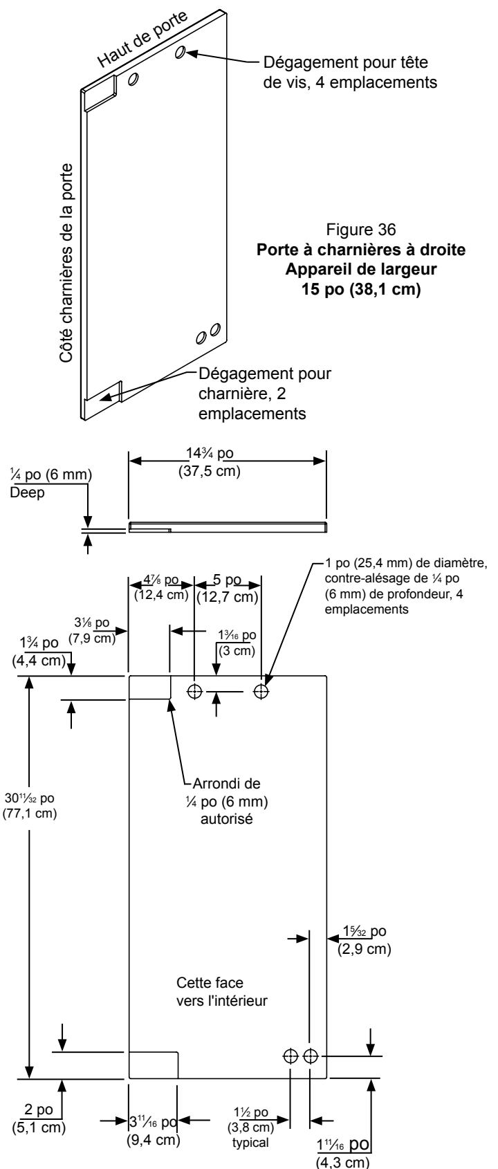
Figure 37 Porte à charnières à droite Appareil de largeur 15 po (38,1 cm)
