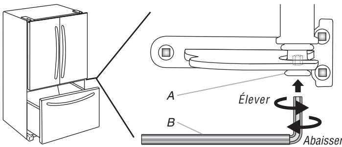
A. Axe de charnière inférieure B. Clé à tête hexagonale de ⅛"
