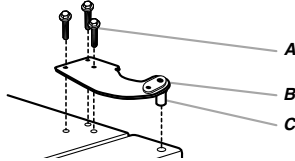
A. Vis de charnière à tête hexagonale de \frac{5}{16} " B. Charnière supérieure C. Axe de charnière
