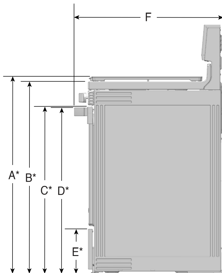
VUE LATÉRALE
