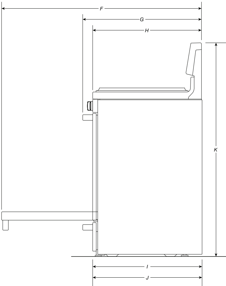
VUE LATÉRALE
