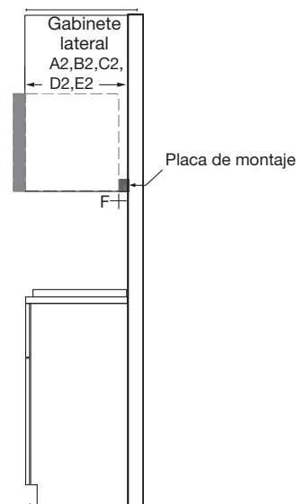
VISTA LATERAL
