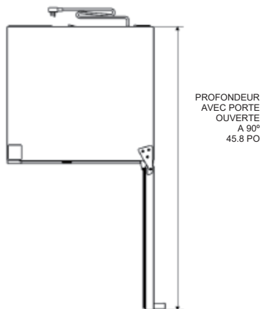
HAUT DU CENTRE DE BREUVAGES AVEC PORTE OUVERTE A 90°
