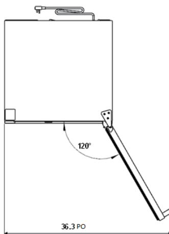
HAUT DU CENTRE DE BREUVAGES AVEC PORTE OUVERTE A 120°
