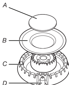
Brûleur à double flamme A. Chapeau interior B. Chapeau exterior C. Répartiteur D. Électrode
