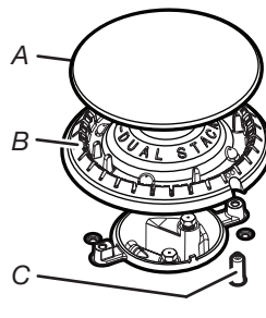
Brûleur double A. Chapeau B. Répartiteur C. Électrode
