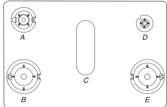
A. Mediana (Semirápido) B. Grande (Ultrarápido) C. Oval (Ovalado) D. Pequeña (Auxiliar) E. Grande (Ultrarápido)
