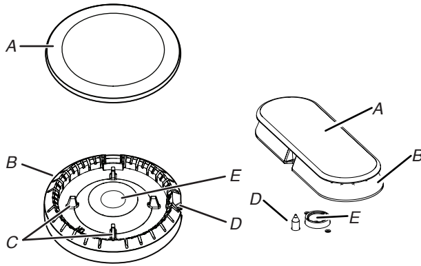
A. Tapa del quemador B. Base del quemador C. Espigas de alineación D. Encendedor E. Abertura del tubo de gas
